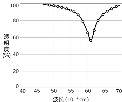
图 23.6: 通过一个薄氯化钠膜 ( 0.17 \mu m ) 的红外辐射透射
